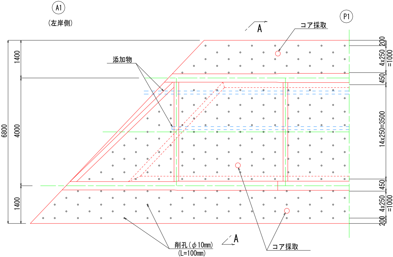
桁下面図
