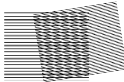
モアレの例
