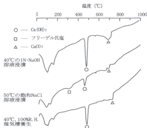
図-6 コンクリートの DSC 曲線 (安山岩碎石, 浸漬期間: 13 週)
