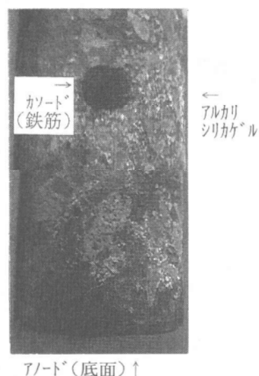
写真-3 アルカリシリカゲルの生成状況
