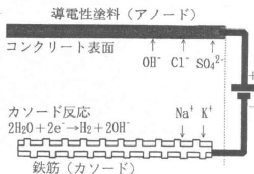
図-4 電気防食のASRに及ぼす影響
