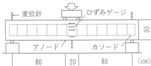
図-1 コンクリート梁試験体の曲げ載荷試験の概要
