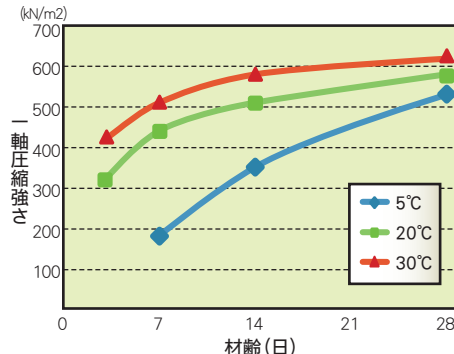
長期強度の測定例(湿潤密度0.6)
