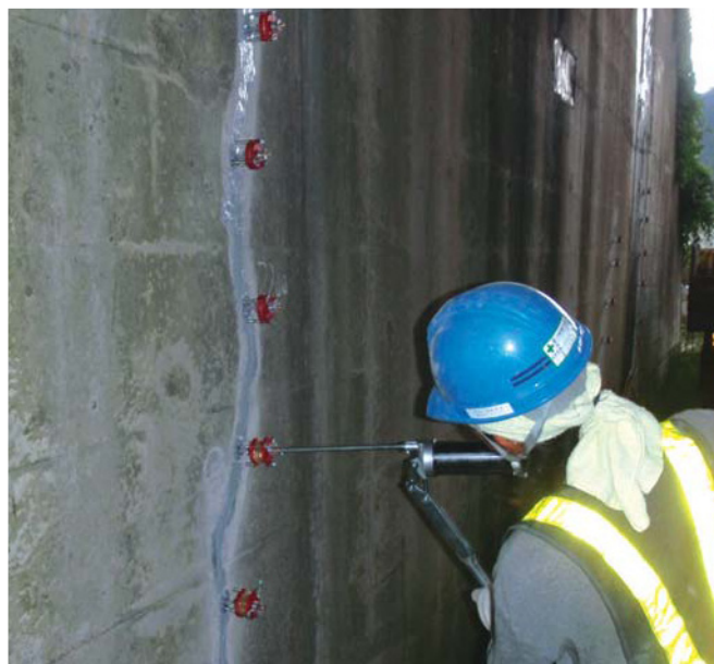
▲クラックボンド注入器を用いた注入補修状況
