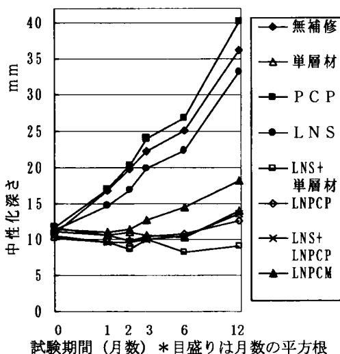
図2 促進中性化試験結果
