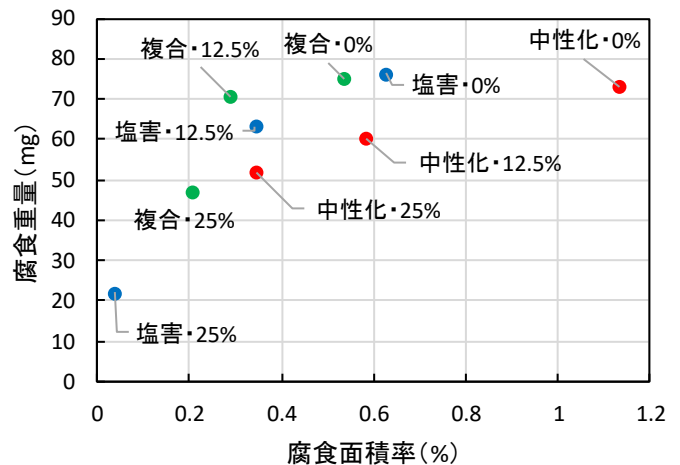
図-4 腐食重量と面積率の関係
