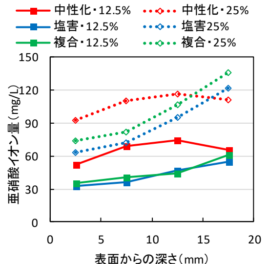
図-3 亜硝酸イオン量の分布
