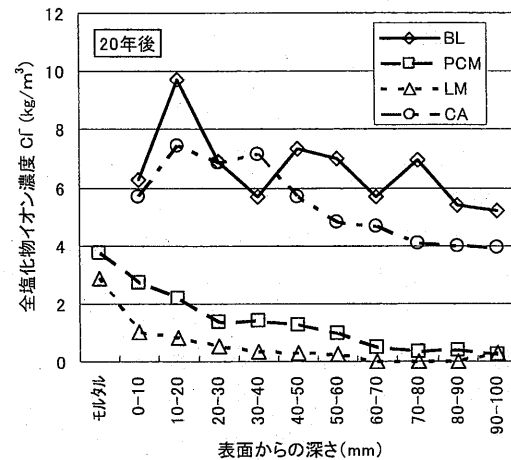
図-7 塩化物イオン濃度分布状況
