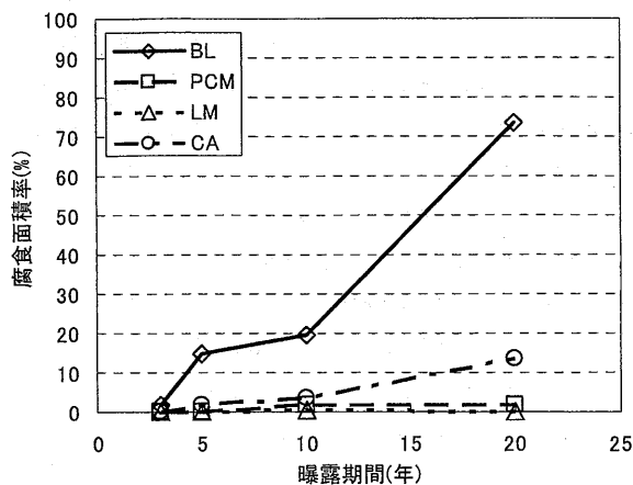
図-12 鉄筋の腐食面積率の経年変化
