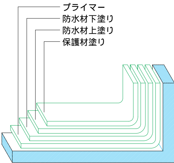
(GRG工法) 地下防水仕様
