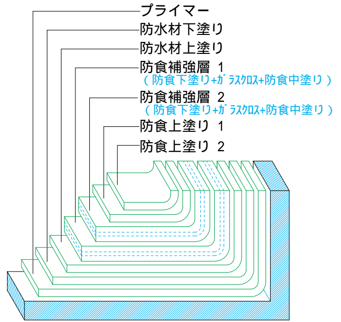
(GR-D工法) 地下防水仕様 (下水エポキシ防食工法)
