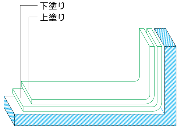
(GA-2工法) 地下防水仕様
