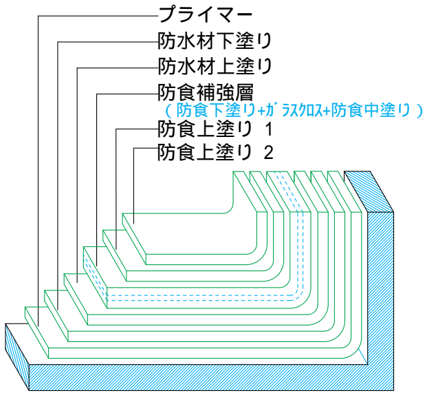
(GR-C工法) 地下防水仕様 (下水エポキシ防食工法)
