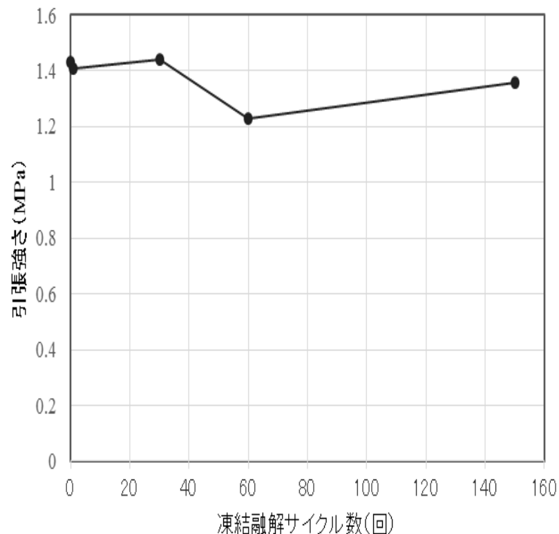
図-1 凍結融解サイクルと引張強さの関係
