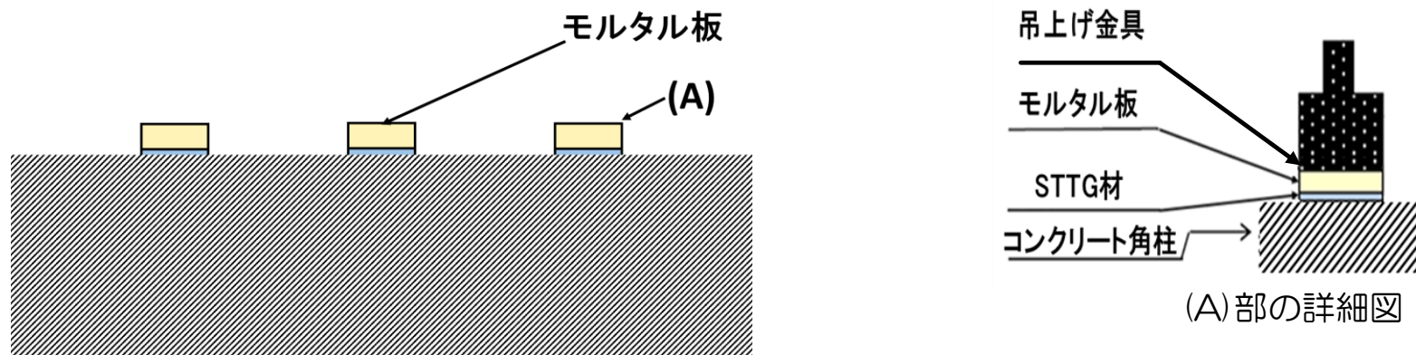
図一2 モルタル板への吊上げ金具の取付け
