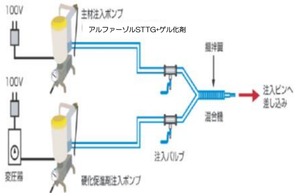
図-1 STTG工法機器構成の概要
