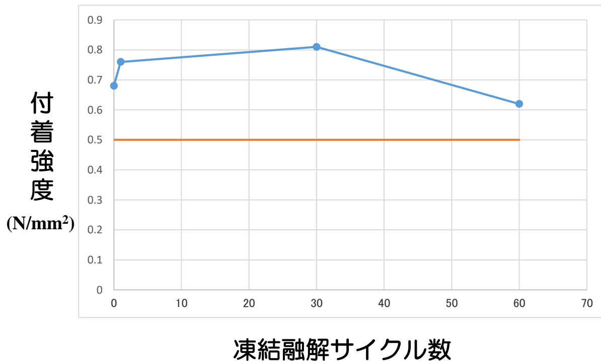
図-3 凍結サイクル数と付着強度との関係
