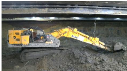
地上走行式ショベル
