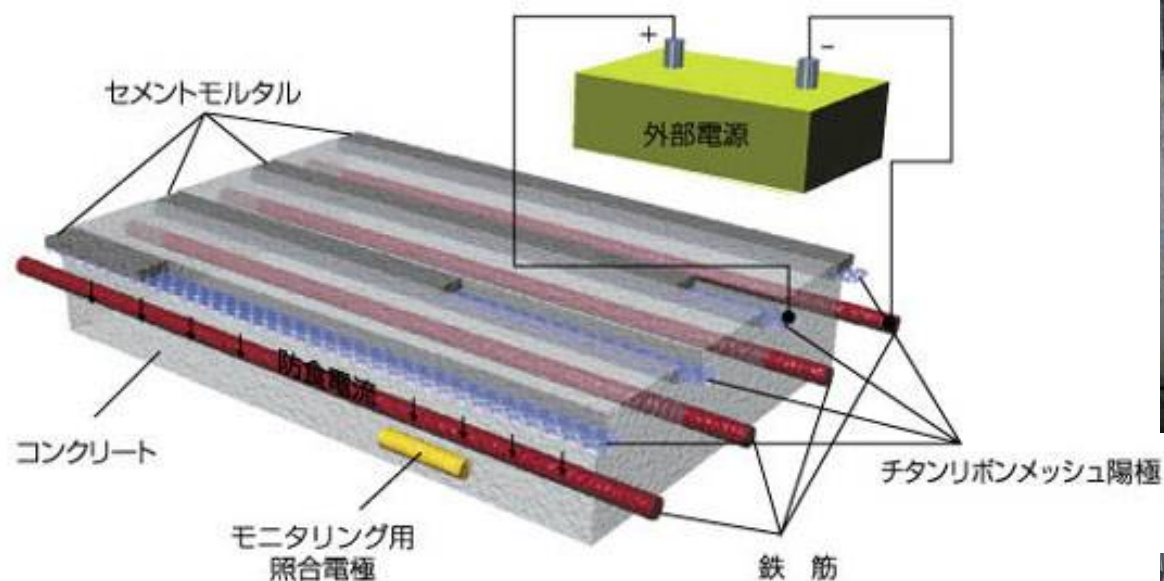
コンクリート表面に溝を切削し陽極を埋設する方式
