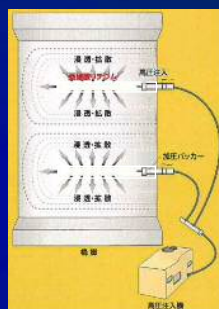
亜硝酸リチウム内部圧入工施工状況
