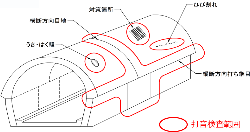
▲ 二回目以降の打音検査の範囲イメージ図
