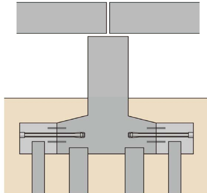
【橋脚基礎の拡幅】
