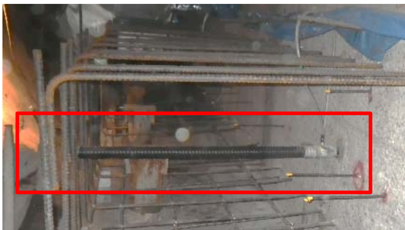
【シース配置】(増フーチング側)
