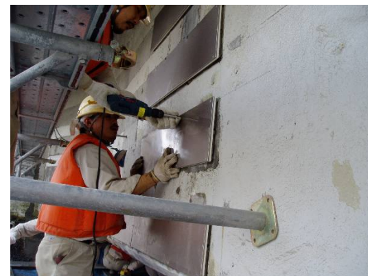
チタントレイの固定
