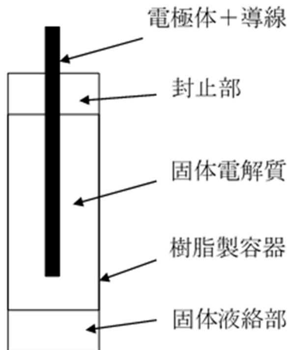
照合電極の基本構造
