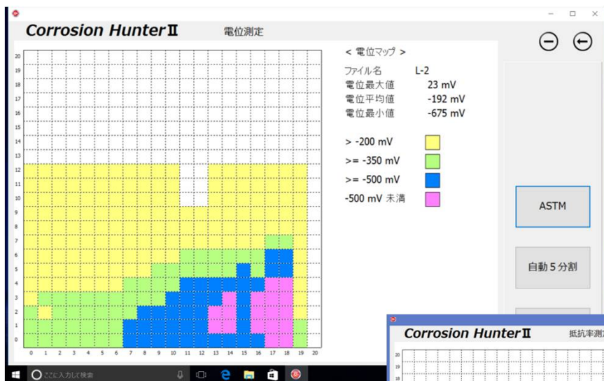
電位測定画面
