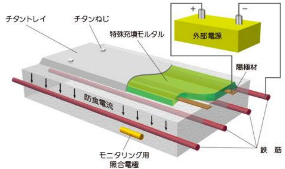
チタントレイ方式の概要
