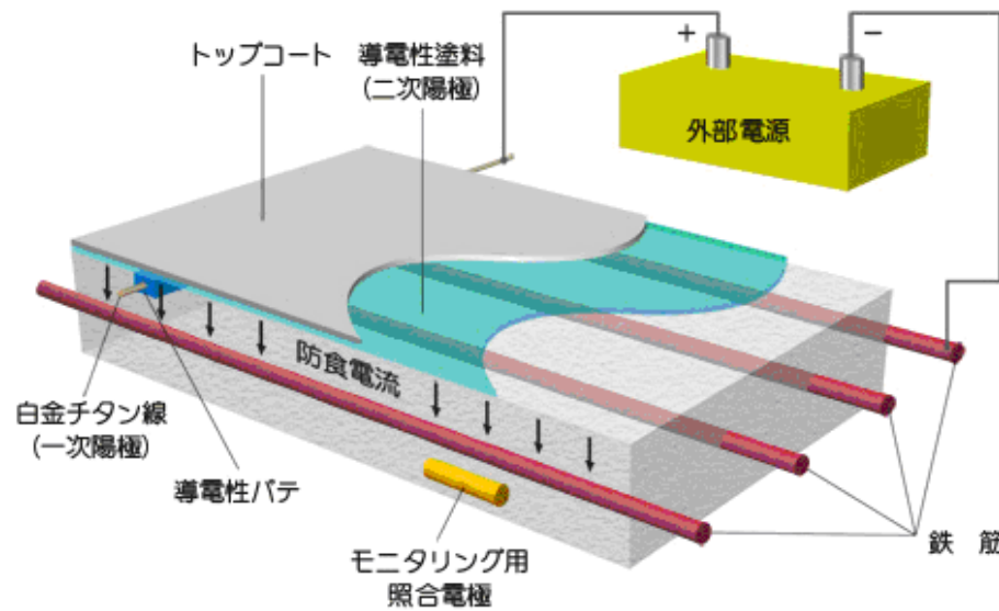
キャプロンコート(導電性塗料)方式の概要
