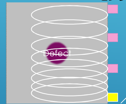
【表面波トモグラフィ】
