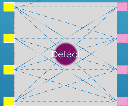
【弾性波トモグラフィ】
