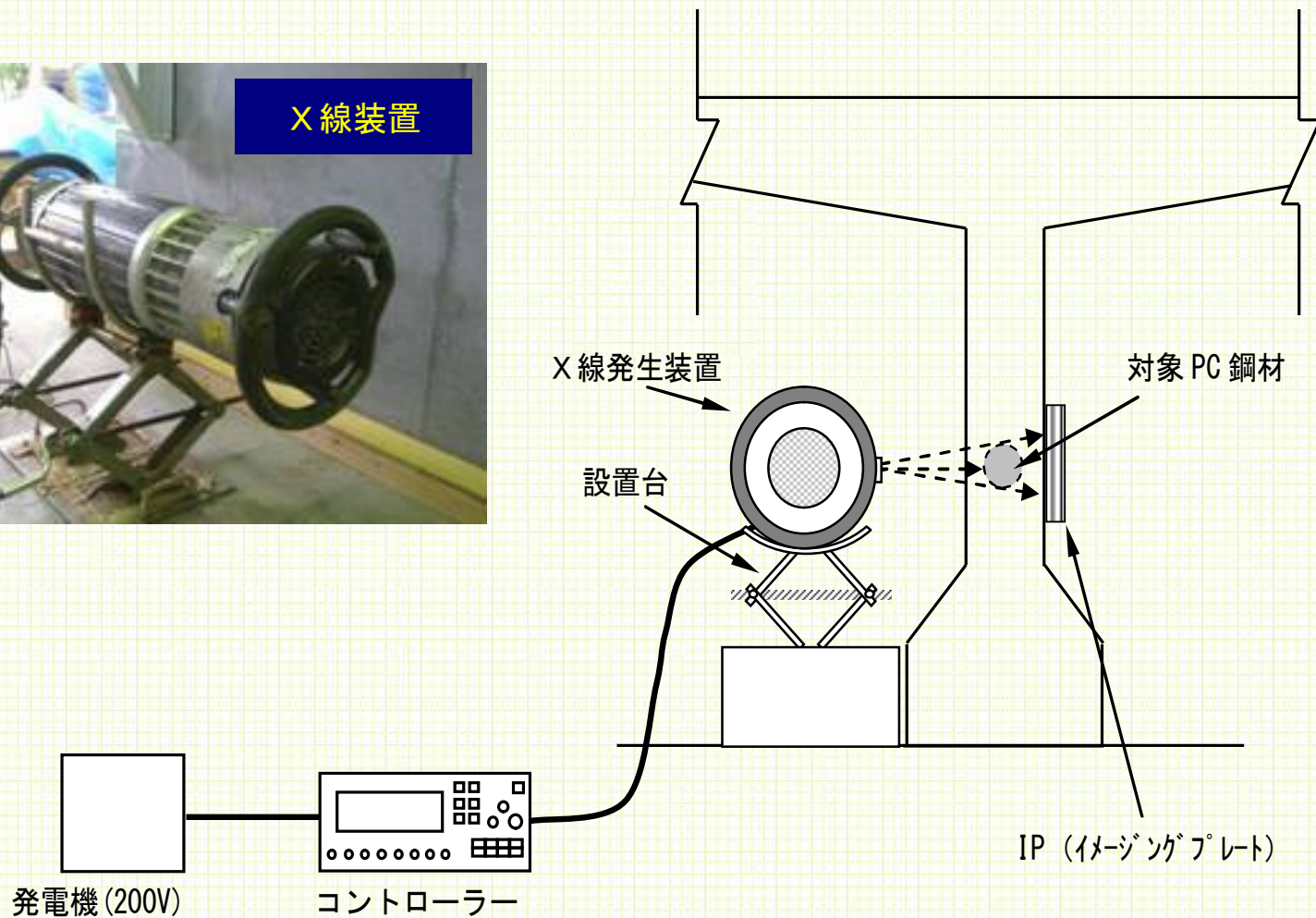
X線透過法概念図
