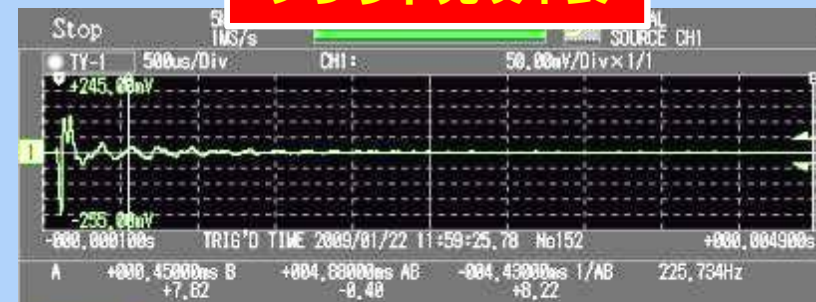
グラウト充填不良
