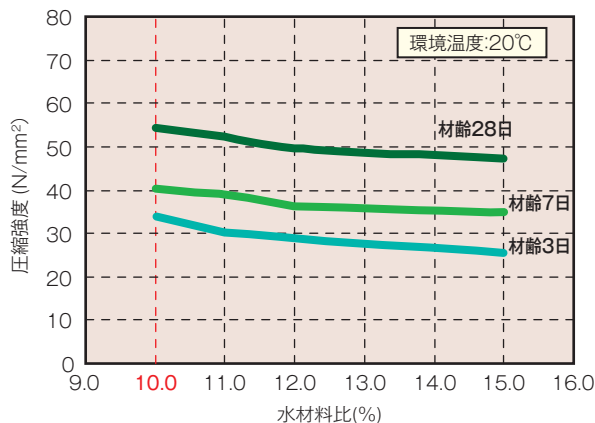
水材料比と圧縮強度の関係
